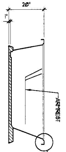
SCALE: 1/2" = 1'-0"
